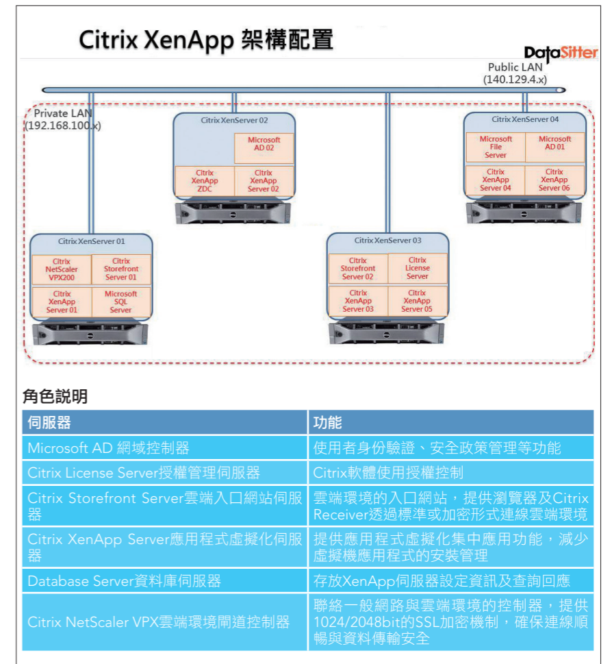
▲大同大學Citrix XenApp架構配置示意圖。
