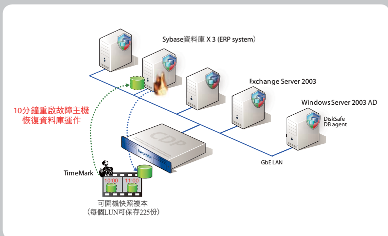
久津實業 CDP 資料保護系統架構圖
